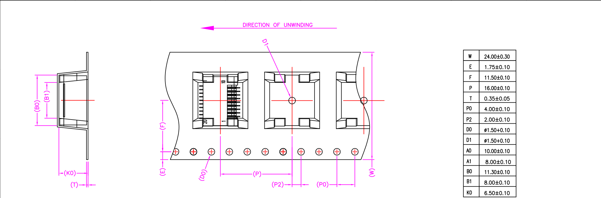
VIEW A-A
