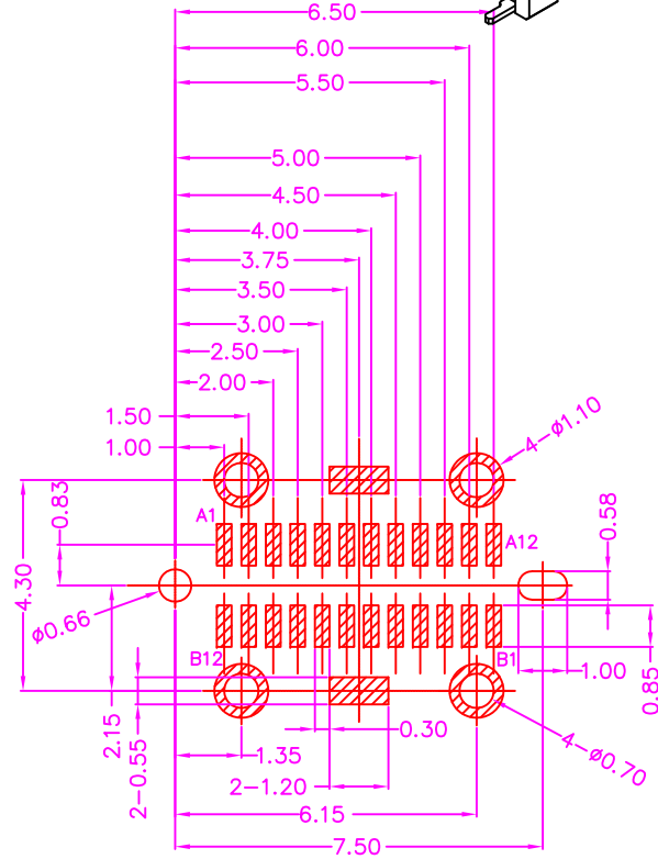
P.C.B. LAYOUT TOP VIEW±0.05 SCALE: 2:1
